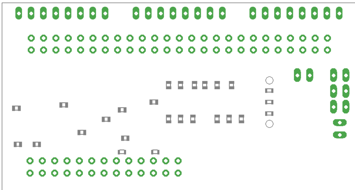
Abbildung 2: Lötseite des ACSI-SCSI-II Adapters
